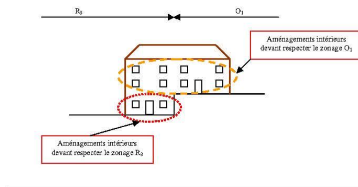
figure 2: exemple d'application du règlement pour les aménagements intérieurs dans le cas d'une rupture importante de la pente talus.
